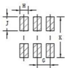
六端产品推荐焊盘尺寸图
