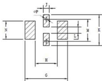
四端产品推荐焊盘尺寸图
