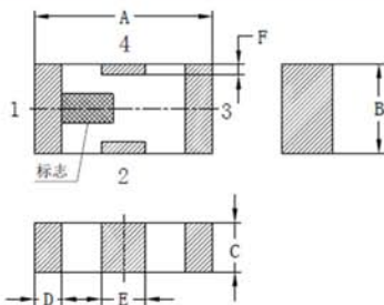
四端产品外形结构
