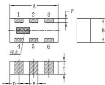
六端产品外形结构
